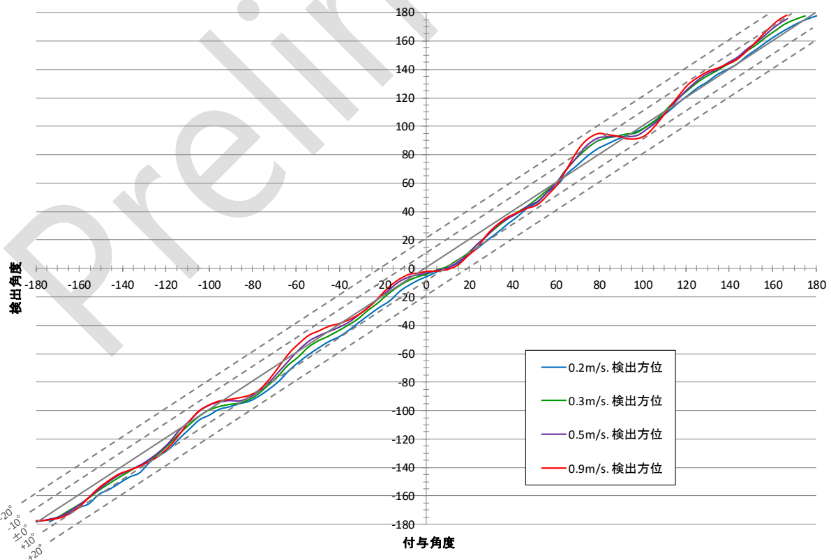
0-1.0m/s.風速域 水平方位検出性能
