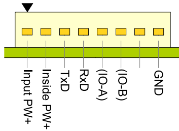
メインインターフェース ピンアサイン図
